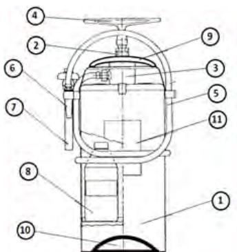
Слика бр. 29. Состав на апаратот брентача
