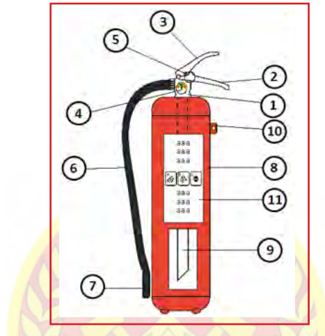
Слика бр. 31. ПП-апарат од типот „S-9“
