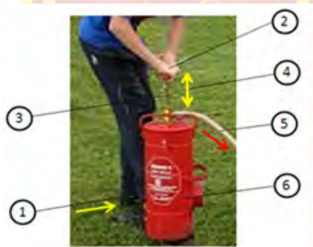
Слика бр. 30. Начин на работа со брентача
